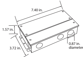
4N1-60W-24V
