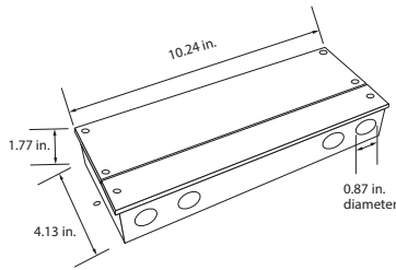
4N1-200W-24V
